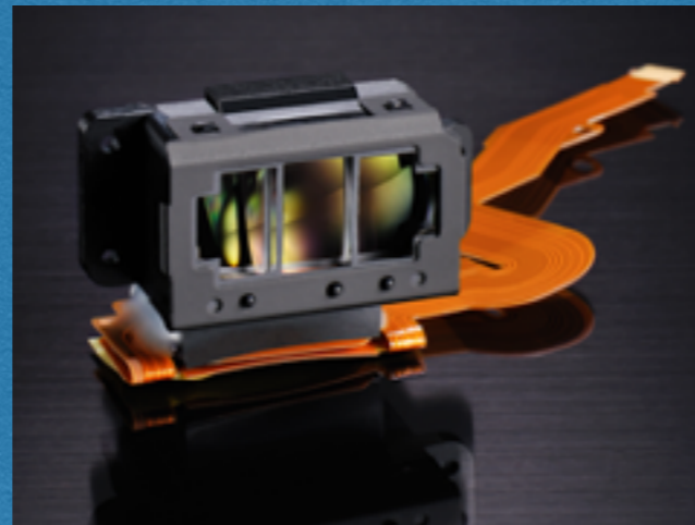
Capteur autofocus CAM3500 d Nikon D800 et D4: 35000 récepteurs
